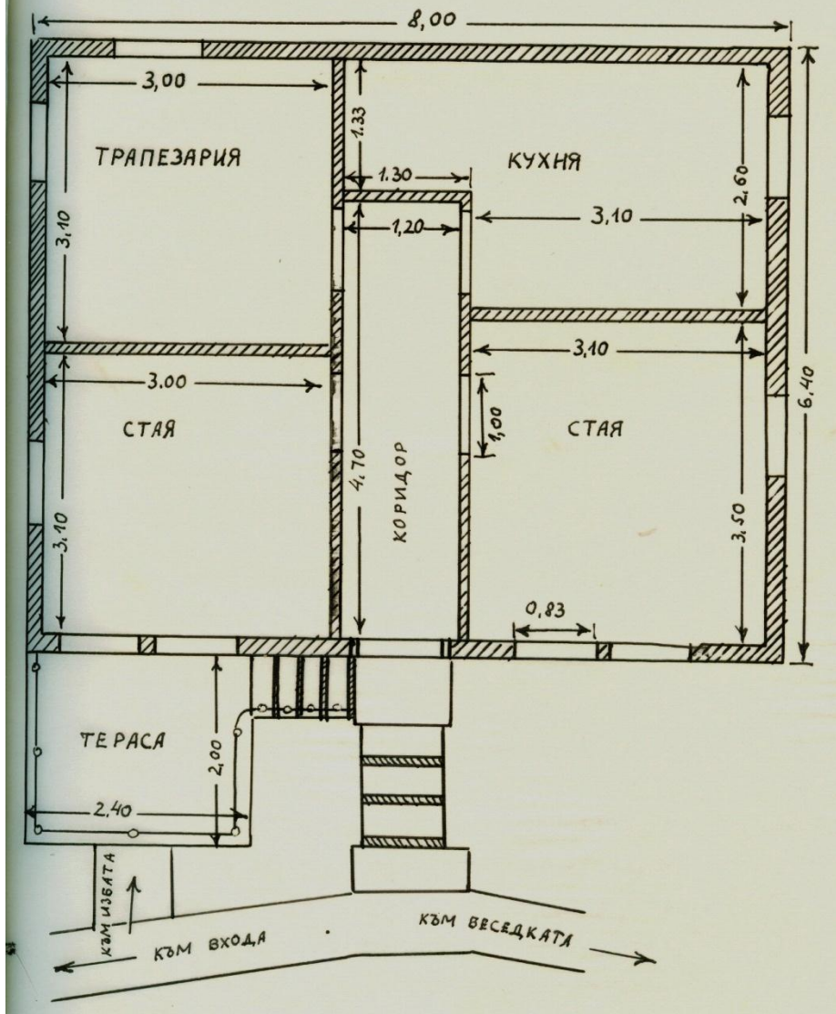
План на етаж на къщата
